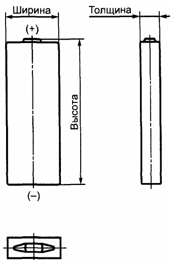
Рисунок 2 - Малогабаритный призматический аккумулятор
