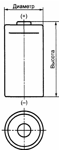
Рисунок 1 - Цилиндрический аккумулятор
